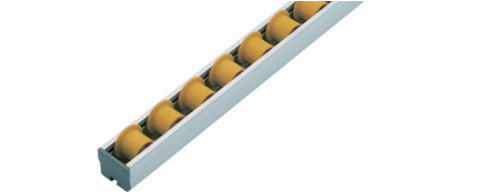
Rullister och hjullister för lättlast
